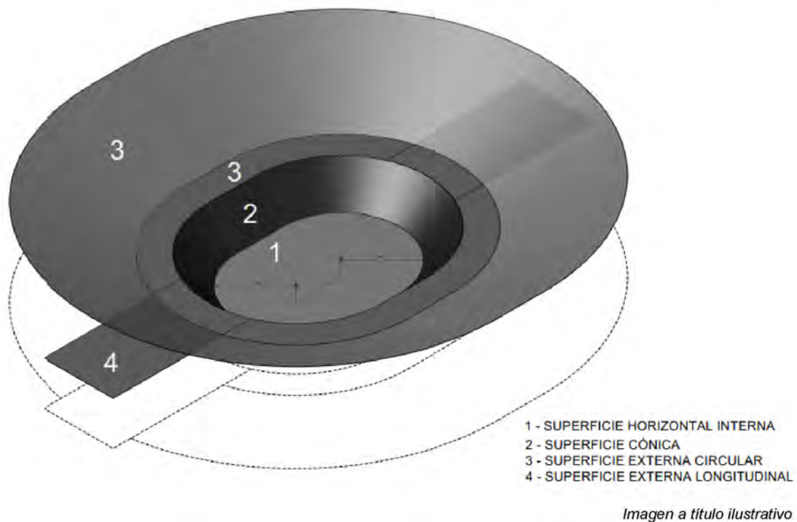
Figura 9: Integración de las superficies horizontal interna, cónica, externa circular y externa longitudinal.
